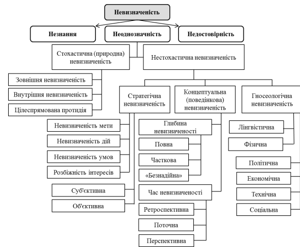
Рис. 2. Схема класифікації різновидів невизначеності
